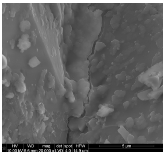
Fig. 6. Piaskowiec kredowy ze złoża Rakowiczki, poddany impregnacji Asolinem OH-30. Widoczne są cienkie powłoki żelowe, z występującymi w ich obrębie krystalitami, pokrywające ziarna. Mikrofotografia SEM
