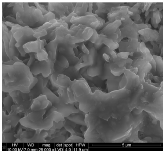
Fig. 5. Piaskowiec kredowy ze złoża Radków, poddany impregnacji Funcosilem KSE 300 E. Widoczne są częściowo krystaliczne formy krzemionki o charakterze gruzłkowym, w nieznacznym stopniu ograniczające porowatość piaskowców. Mikrofotografia SEM
