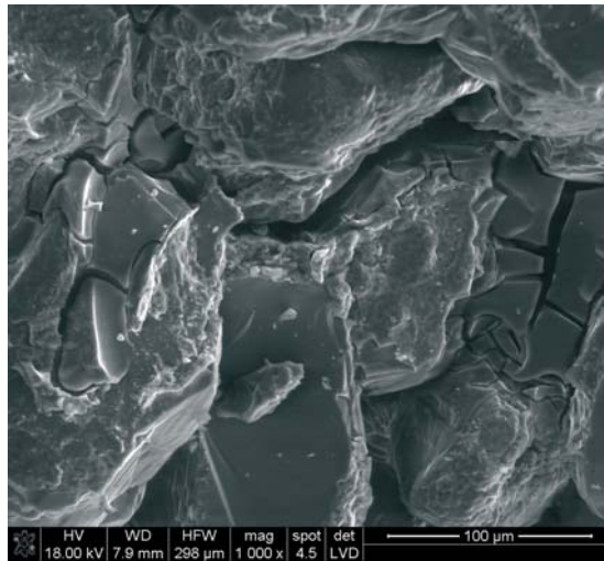
Fig. 9. Piaskowiec kredowy ze złoża Szczytna Zamek, poddany impregnacji Funcosilem KSE 500 E. Pomędzy ziarnami widoczne są silnie spękanе skupienia żelu krzemionkowego. Mikrofotografia SEM
