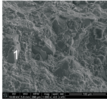
Fig. 25. Obraz skaningowy próbki 1. Widoczne różnej wielkości ziarna czystego kwarcu
